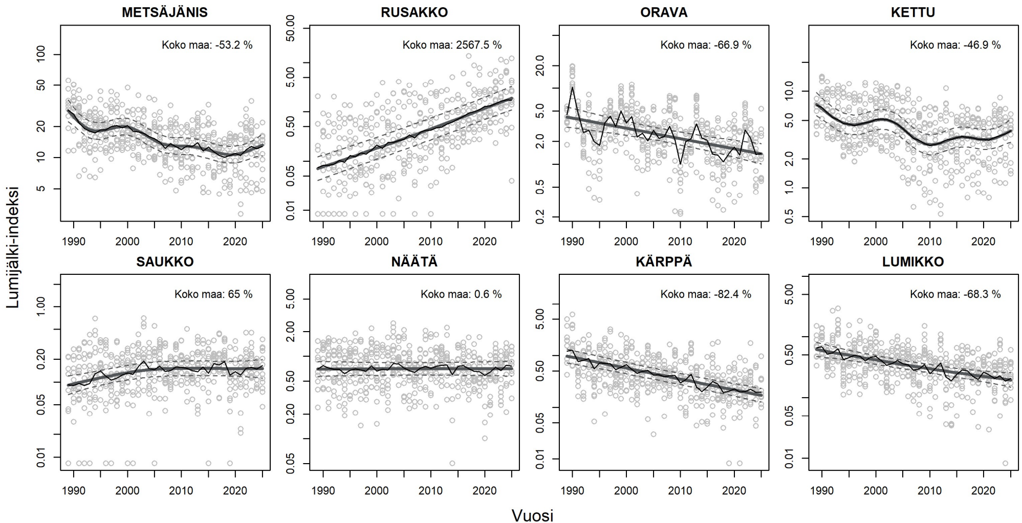
Kuva 1. Lajikohtaiset kannankehitykset koko maassa 1989–2025 riistakolmiolaskentojen perusteella. Ympyrät ovat riistakeskusaluekohtaisia vuosittaisia lumijälki-indekskejä. Paksu viiva osoittaa ajallisen trendin ja katkoviivat rajaavat tälle 95 % luottamusvälin. Kapea musta yhtenäinen viiva näyttää vuosittaiset yhdenmukaiset poikkeavuudet trendistä. Huomaa logaritminen pystyakseli. Lähde: Luonnonvarakeskus.
